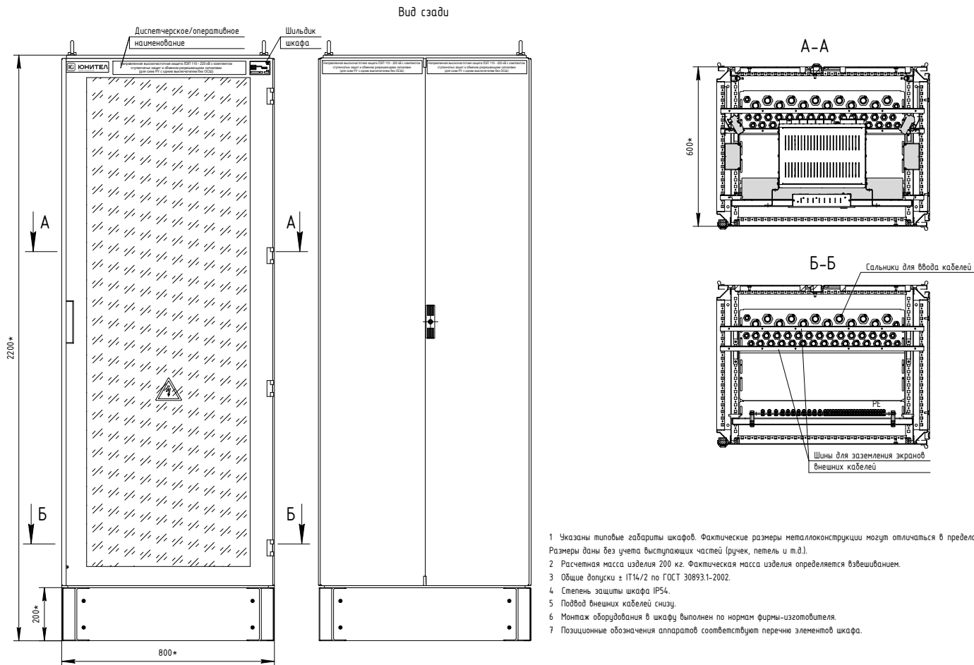
Рисунок В.1 – Чертеж общего вида (часть 1)
