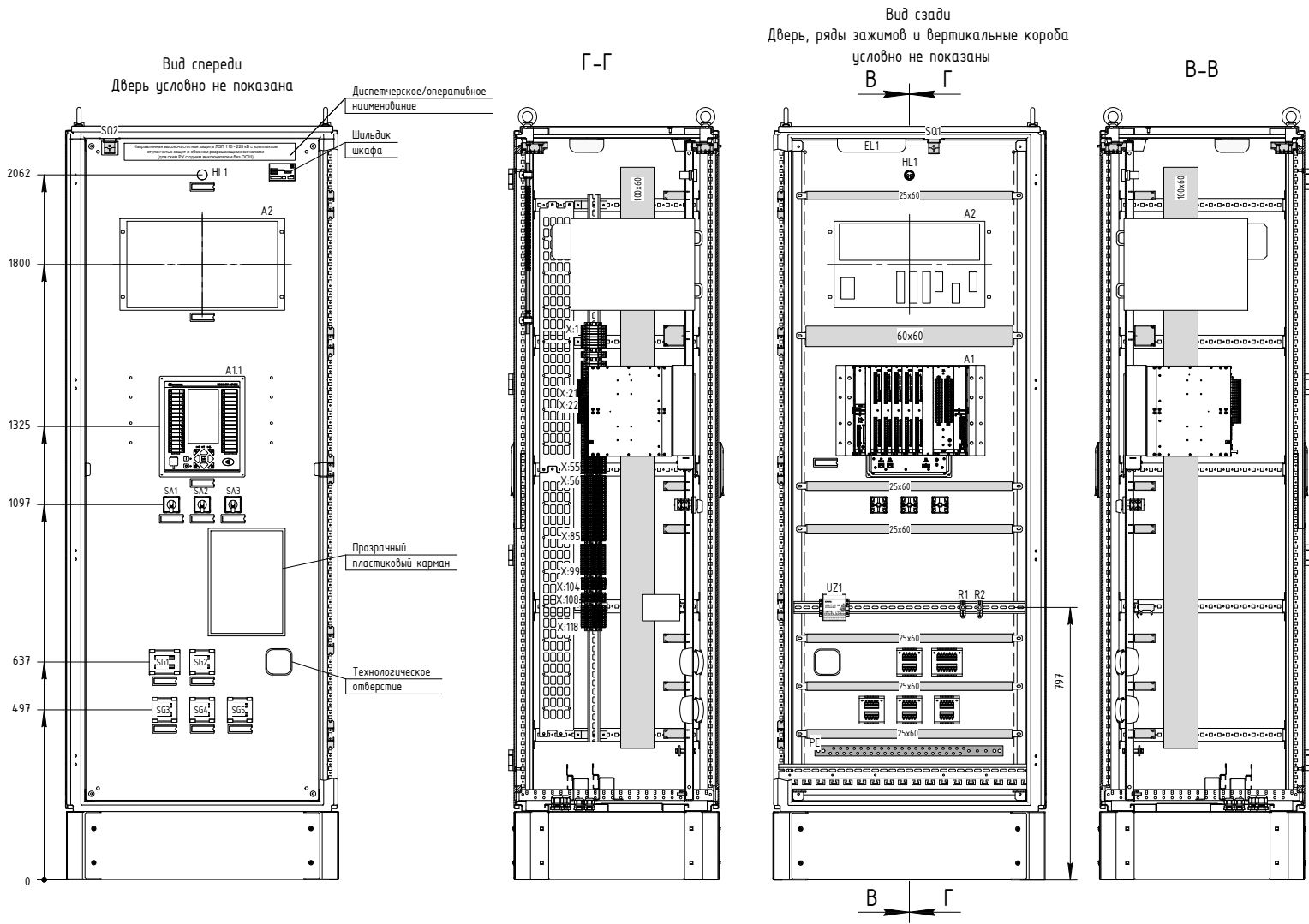
Рисунок В.2 – Чертеж общего вида (часть 2)
