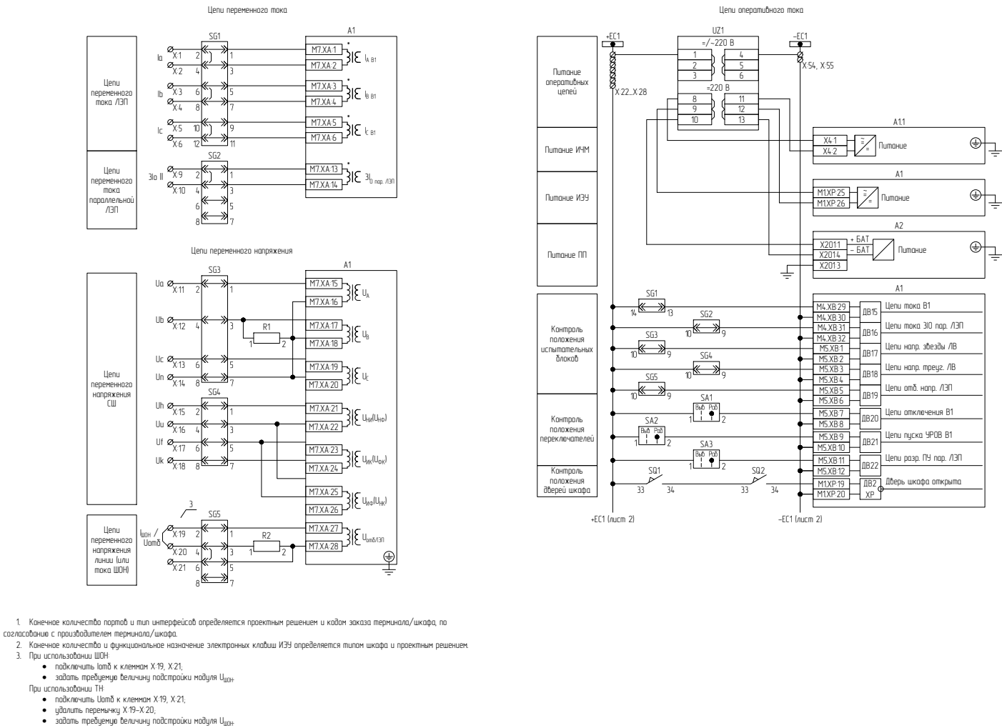
Рисунок Г.1 – Схема электрическая принципиальная (часть 1)
